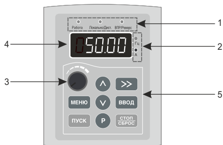
Рисунок 4-1. Панель управления
